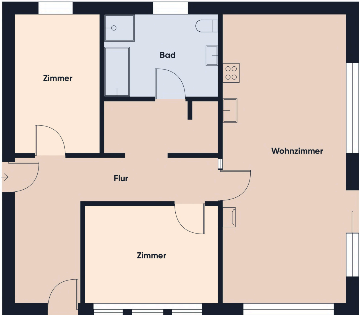
Grundrissplan UG
