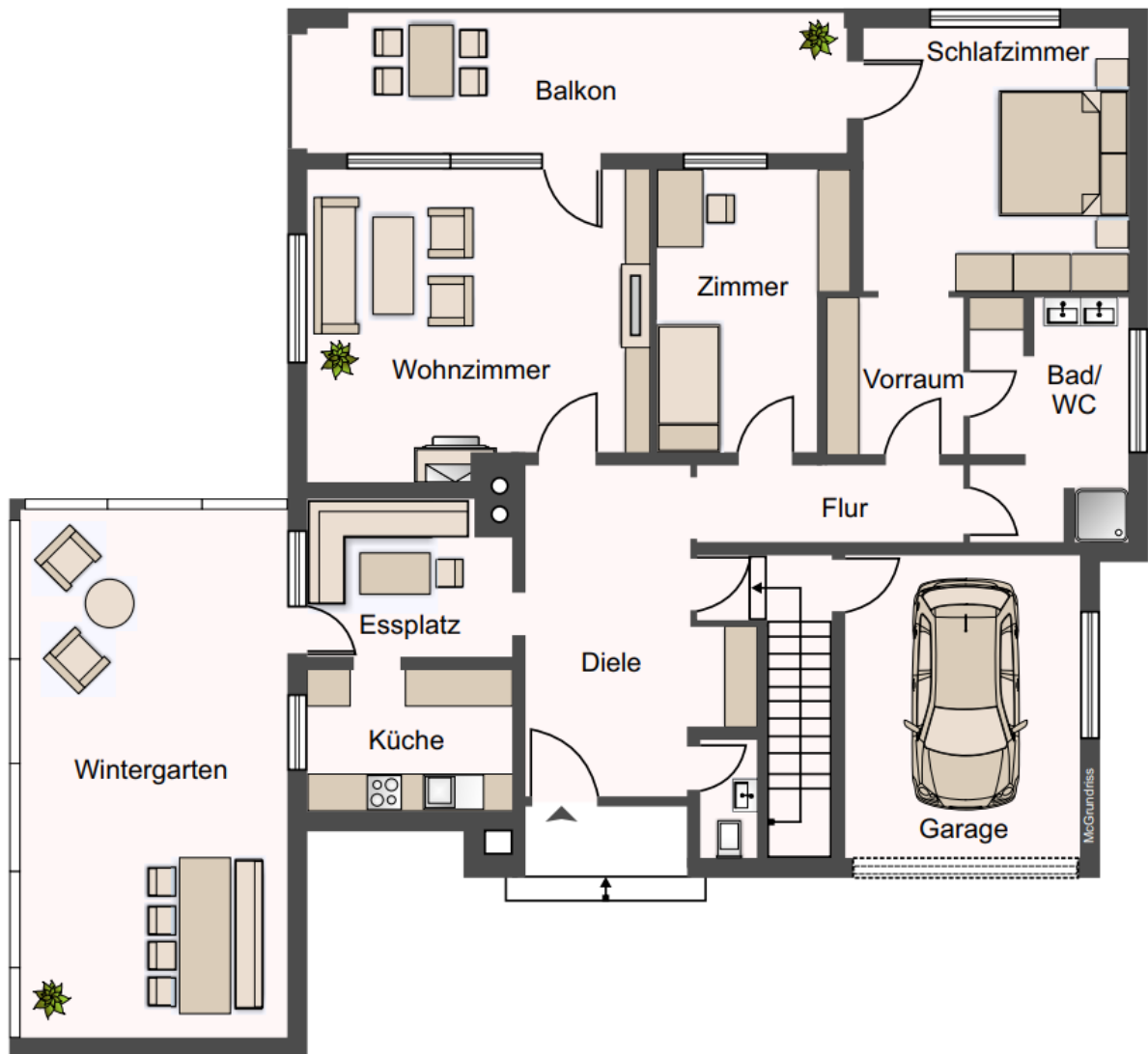
Erdgeschoß
