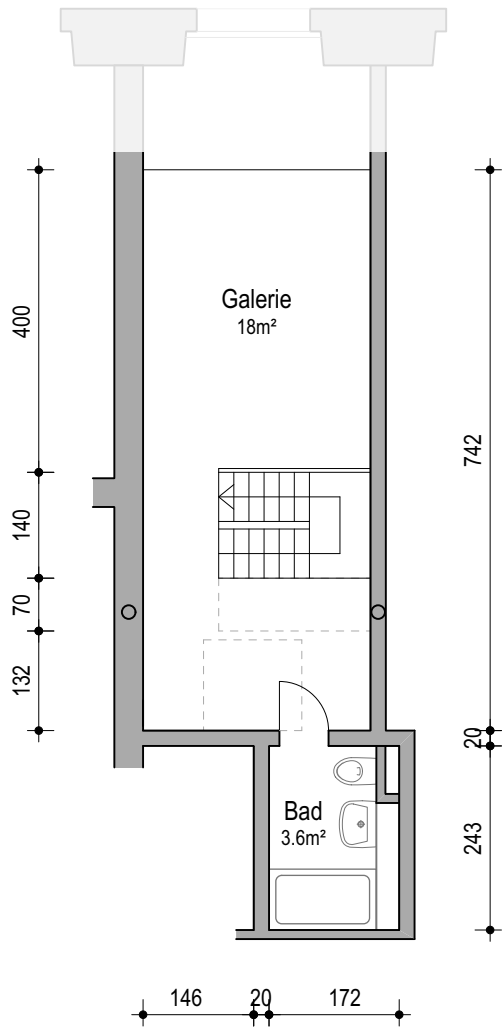
Top F35b Galerie Mst. 1:100
