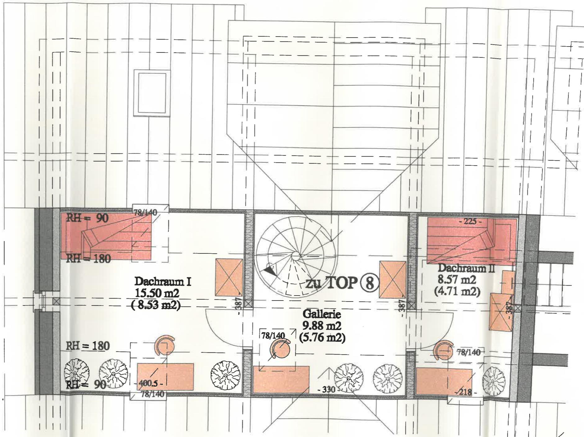
Dachgeschoss-Grundriß
