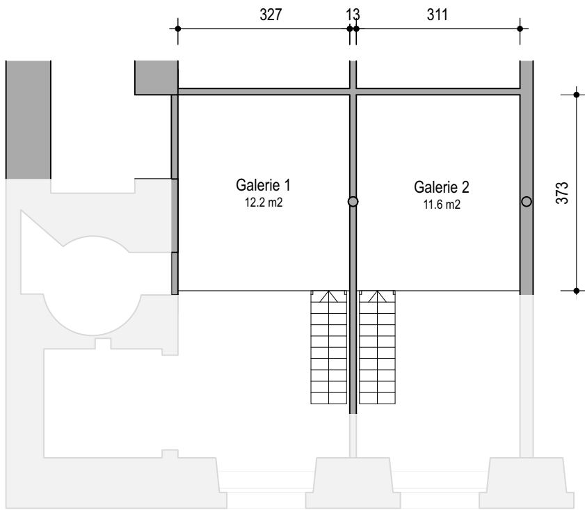
Top F18a Galerie Mst. 1:100
