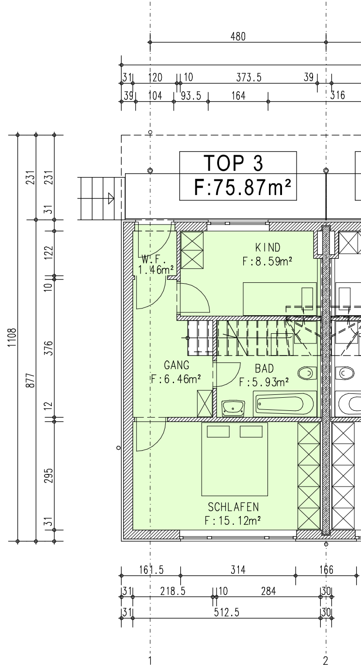
GRUNDRISS 1.OG M1:100
