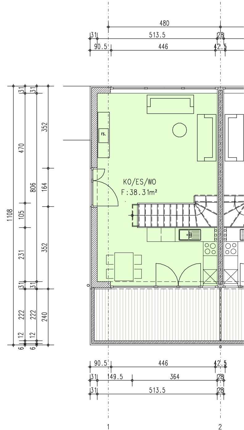
GRUNDRISS DG M1:100
