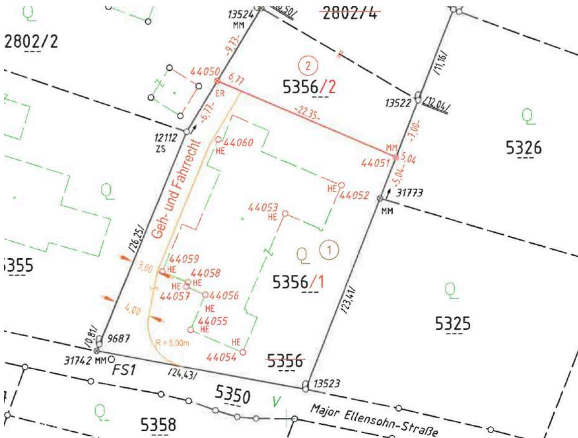
Grundstücksplan mit Geh- u Fahrrecht
