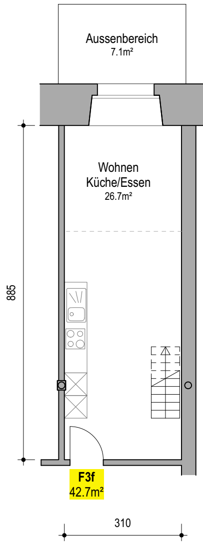
Top F3f Wohnung Mst. 1:100
