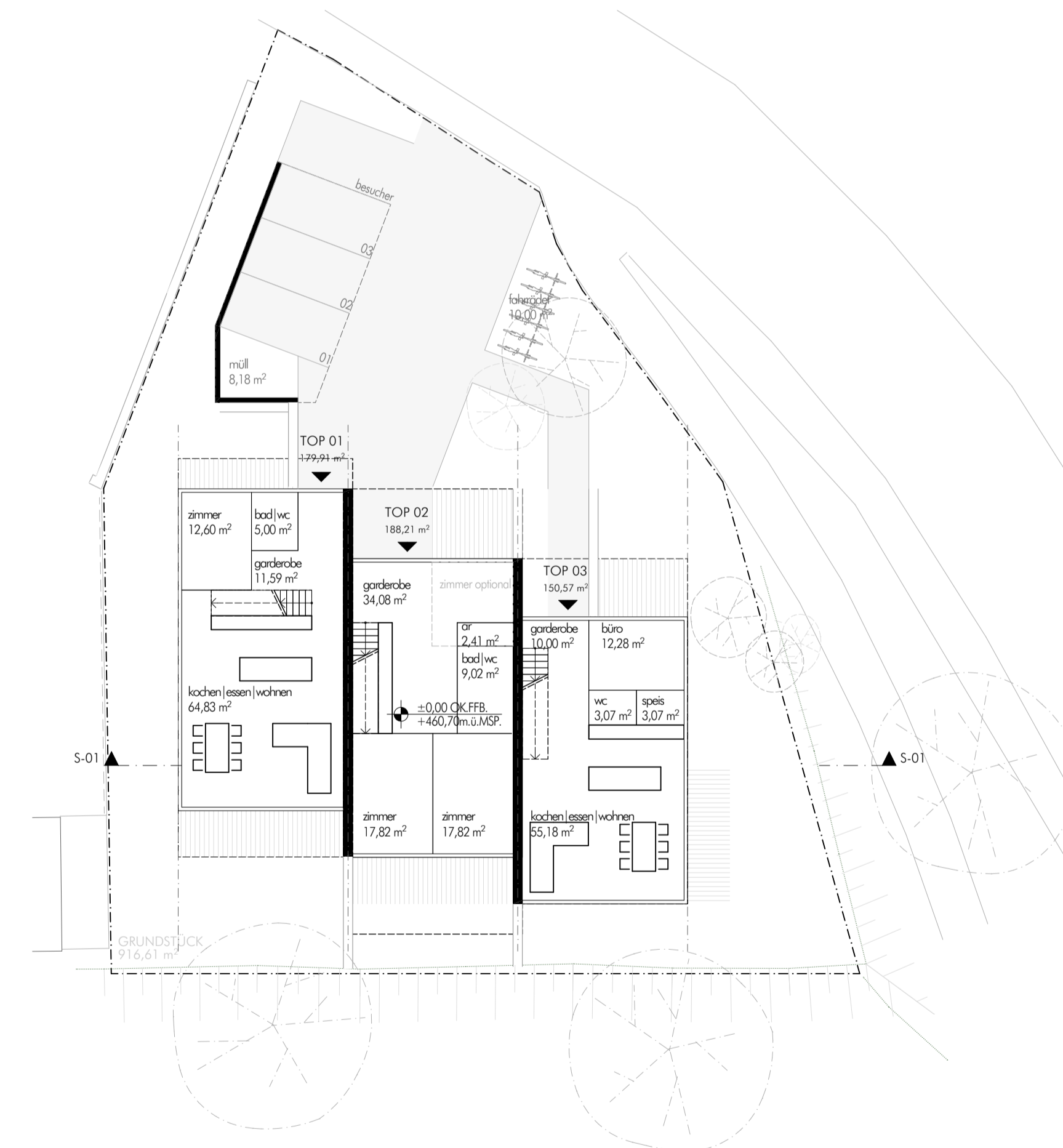
GRUNDRISS EBENE 00
