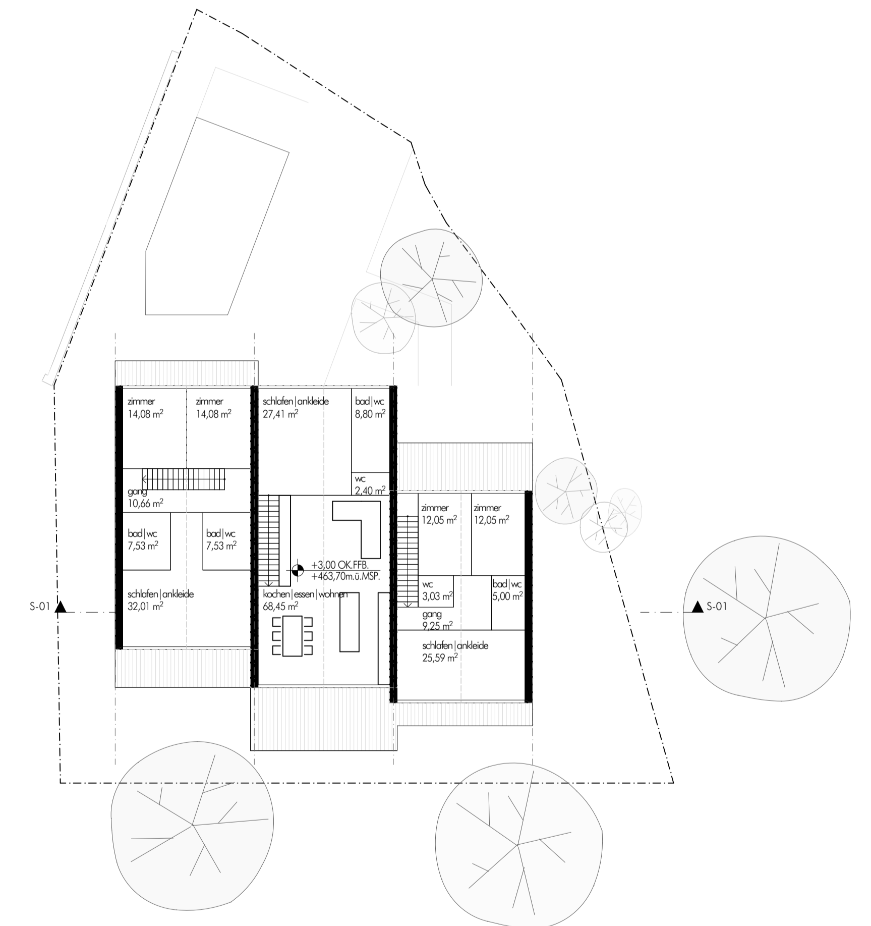
GRUNDRISS EBENE 01
