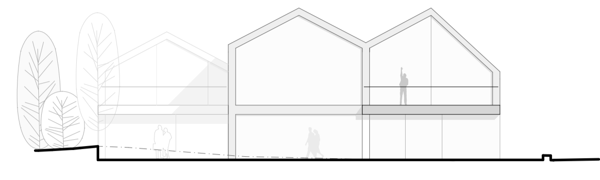
ANSICHT NORD
