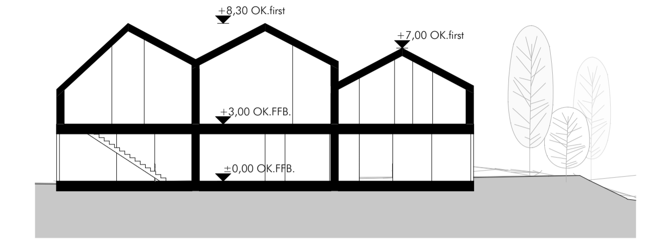
SCHNITT 01
