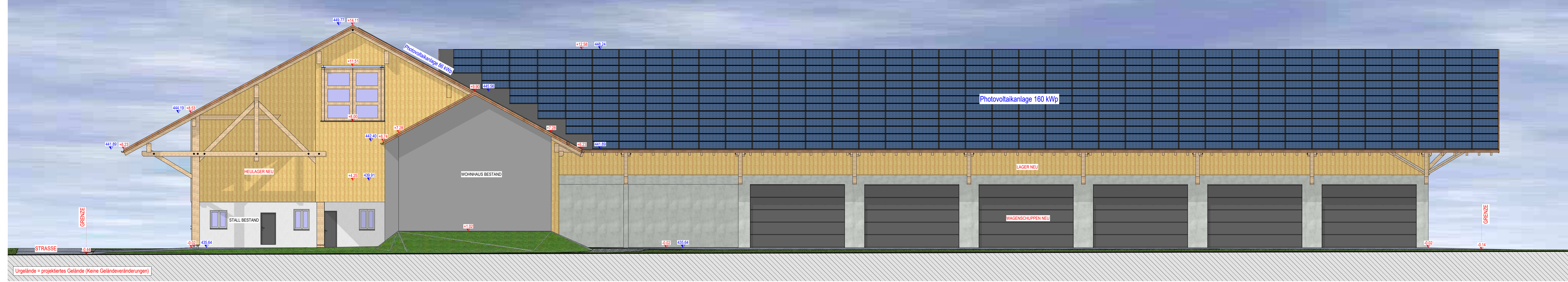
ANSICHT SÜDEN / M 1:100
