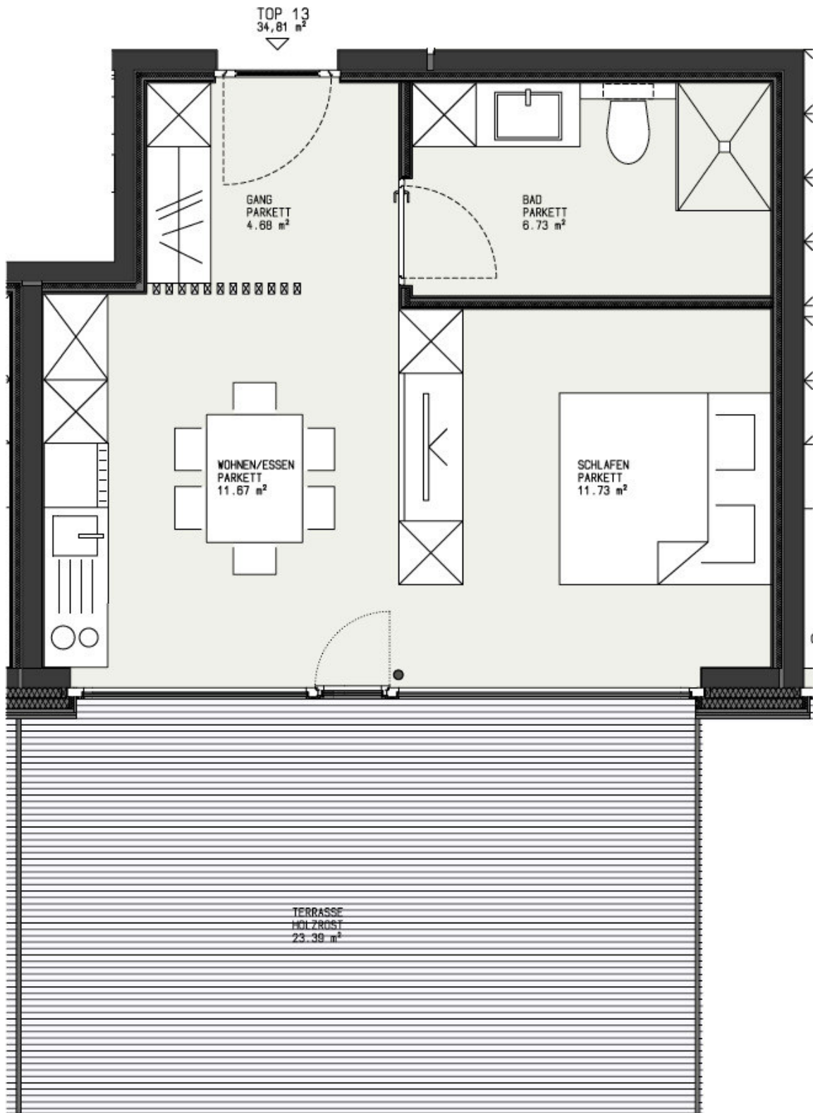
Grundrissplan
